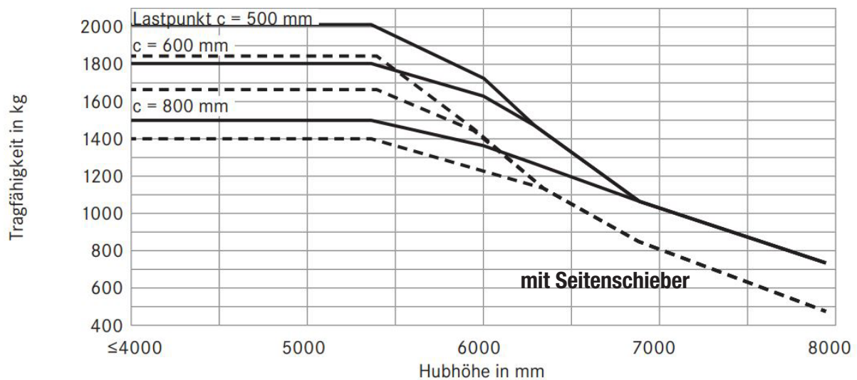
RX 20-20P Dreifach-Hubgerüst Einfach SE-Bereifung
