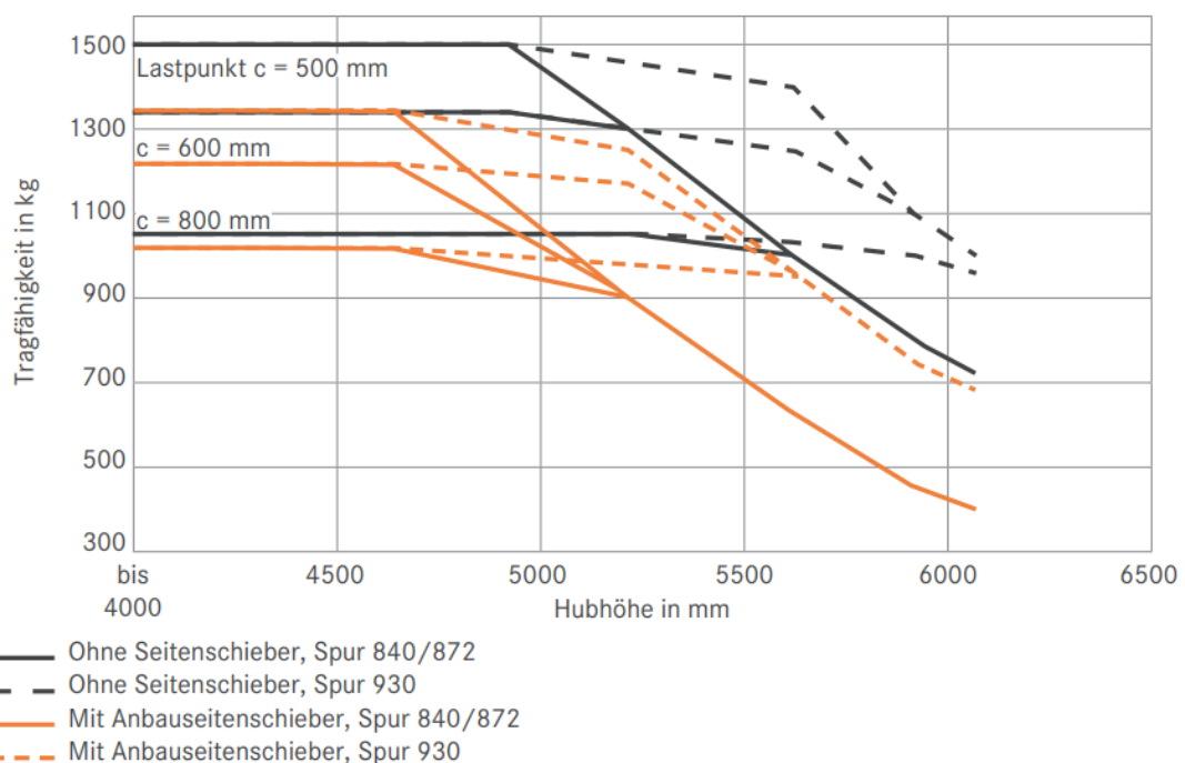
RX 50-15 Dreifach-Hubgerüst Superelastik-Bereifung
