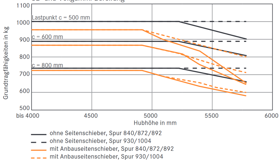
Grundtragfähigkeiten RX 50-10 Dreifach-Hubgerüst SE- und Vollgummi-Bereifung
